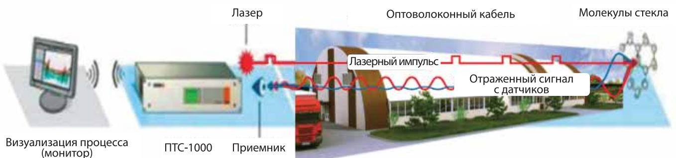
Схема подключения основных компонентов системы ПТС-1000.
